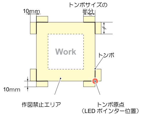
トンボ形状 : Type.5 (フリーモード・円)
