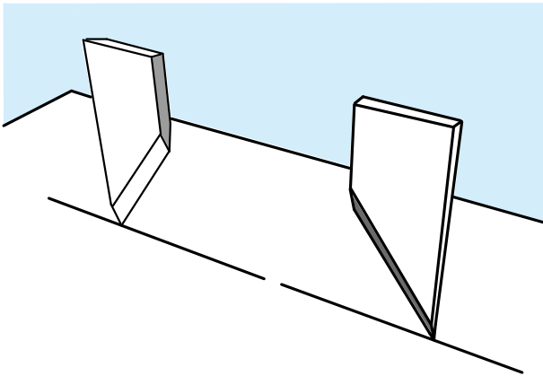
【偏芯 A をマイナスに調整する場合】
