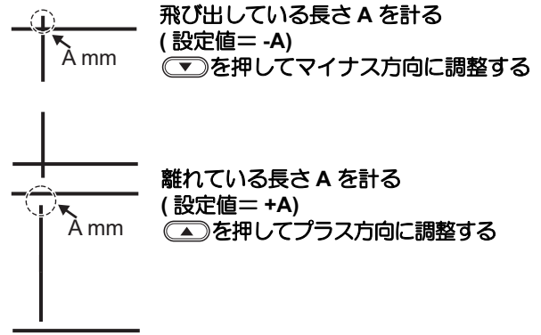
【偏芯 A をプラスに調整する場合】
